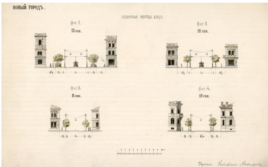
Новый город в Порт-Артуре. Поперечные разрезы улиц. Проект А. Антипова. 1900 г. Ф. 3л. Оп. 37. Д. 11269.
