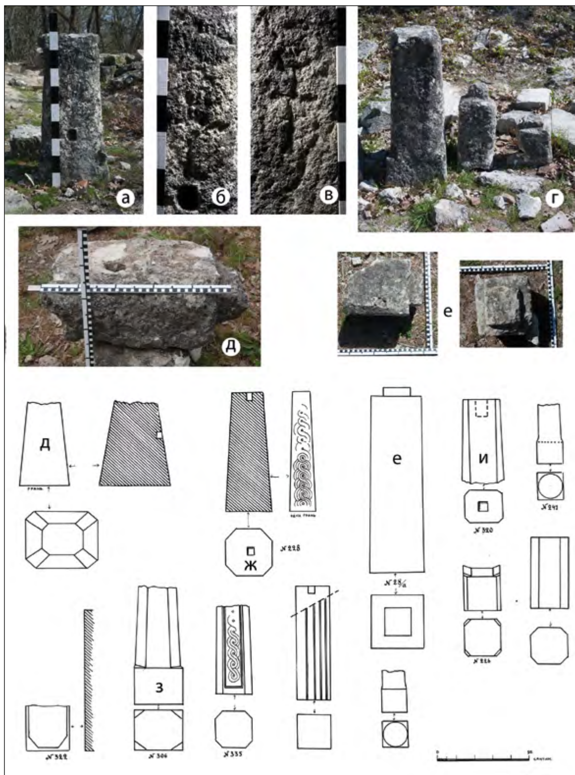
Рис. 3. Архитектурные детали базилики. Вверху – цветные фото автора, внизу — архивный чертёж [РО НА ИИМК РАН. Ф. Р-І. Д. 125. Л. 15]. Буквенные обозначения на чертеже проставлены автором в целях унификации. Описание деталей см. в тексте статьи.
