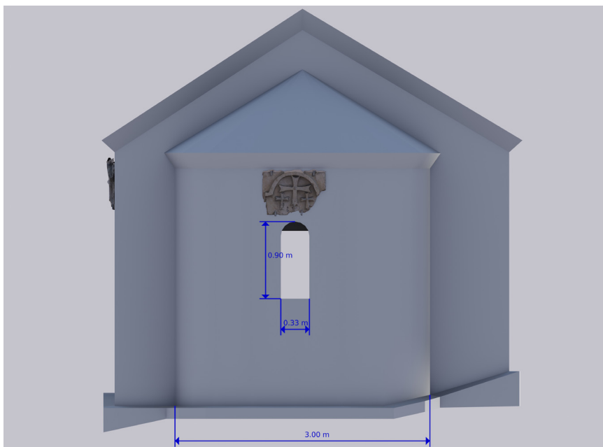
Рис. 7. Восточный фасад Нижней церкви. Реконструкция А. Д. Карнаушенко, Э. Н. Карнаушенко, Л. К. Казеннова, 2023 г.
