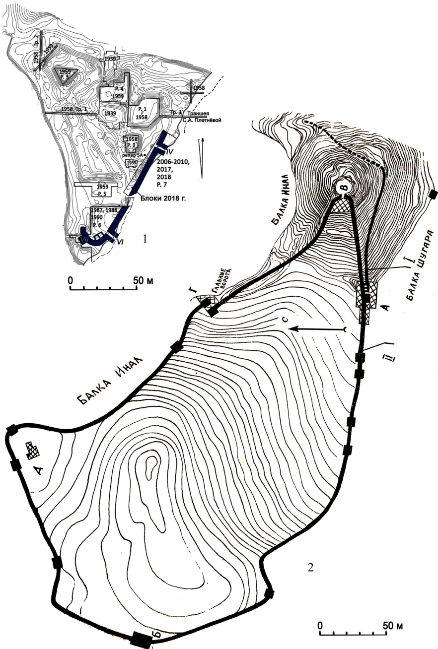
Рис. 1. Крепости Правобережная Цимлянская и Хумаринская: 1 – Правобережная Цимлянская (синим тонированы южная и участок восточной стен с башнями), раскопки 1987–2020 гг. 2 – Хумаринская (по: Биджиев, 1983. Рис. 1).
