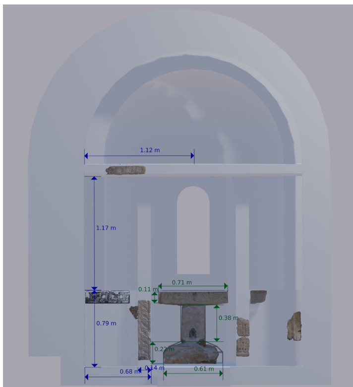
Рис. 12. Алтарная преграда и престол Нижней церкви. Реконструкция А. Д. Карнаушенко, Э. Н. Карнаушенко, Л. К. Казеннова, 2023 г.
