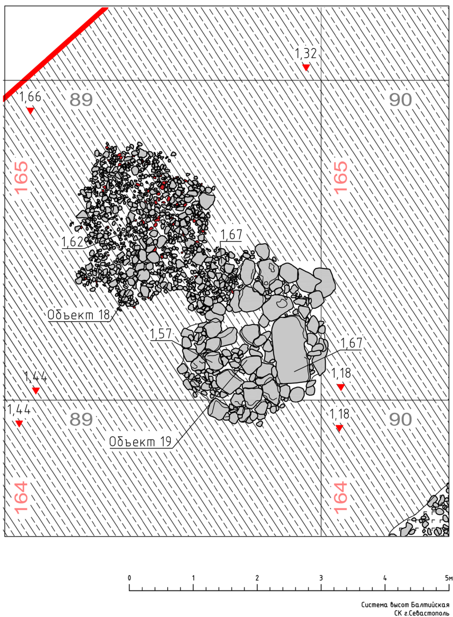
Рис. 2. Общий план объектов 18, 19 раскопа 12.
